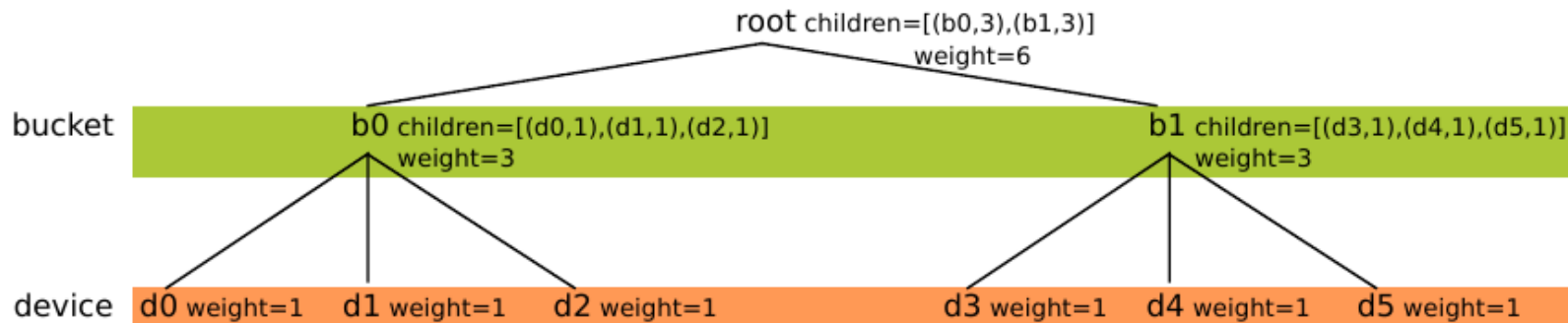
FIGURE 1 – Clustermap utilisé.
