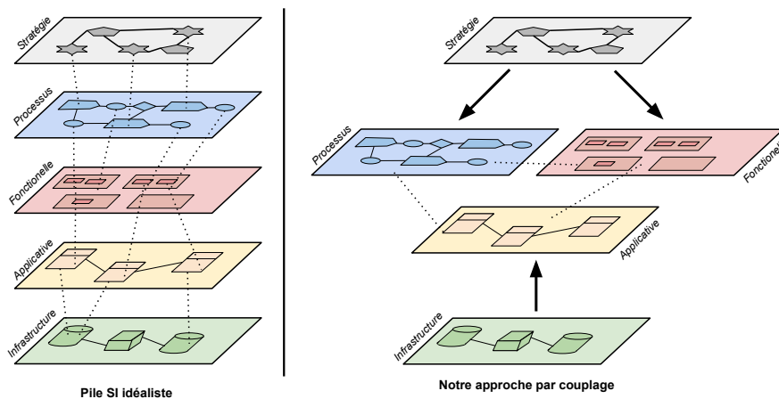
Figure 2. Les couches du SI : la pile idéale et l'aperçu de notre approche
