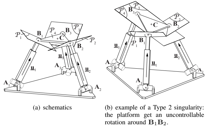
Fig. 3. A 3- UPS robot.
