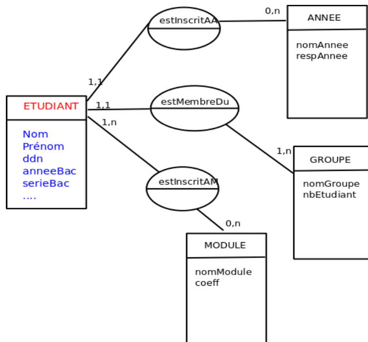
Figure: Un modèle EA du SI gestion IUT
